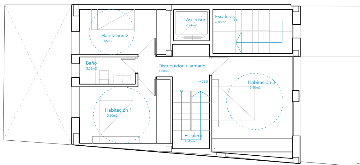
PLANTA PRIMERA Superficie construida: 66,85m² Superficie ocupada: 63%
