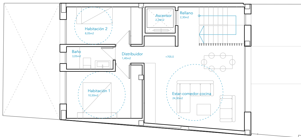
VIVIENDA 2 Superficie útil cerrada: 63,30m² + Ascensor Superficie patio delantero: 5,80m² Superficie cubierta: 52,50m²
