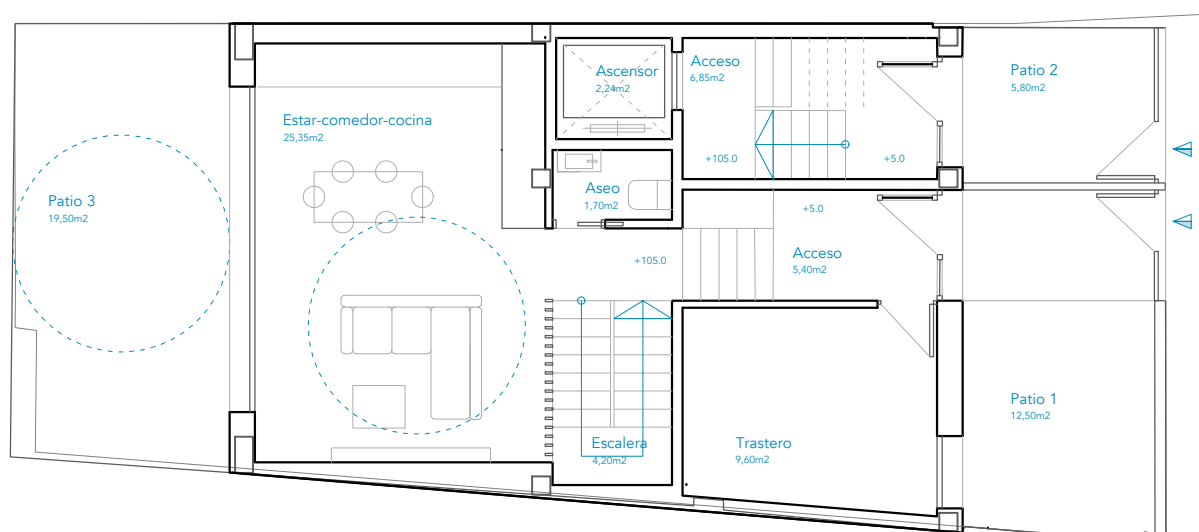
VIVIENDA 1 Superficie útil cerrada: 88,25m² Superficie útil patio delantero: 12,50m² Superficie útil patio trasero: 19,50m²
